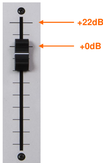
Detalle calibración fader 100mm
