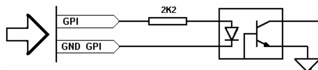
Detalle de la electrónica asociada a la entrada de propósito general por optoacoplador
